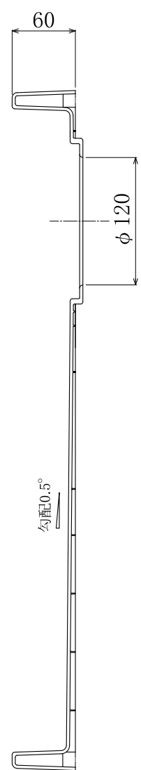
A-A'断面
